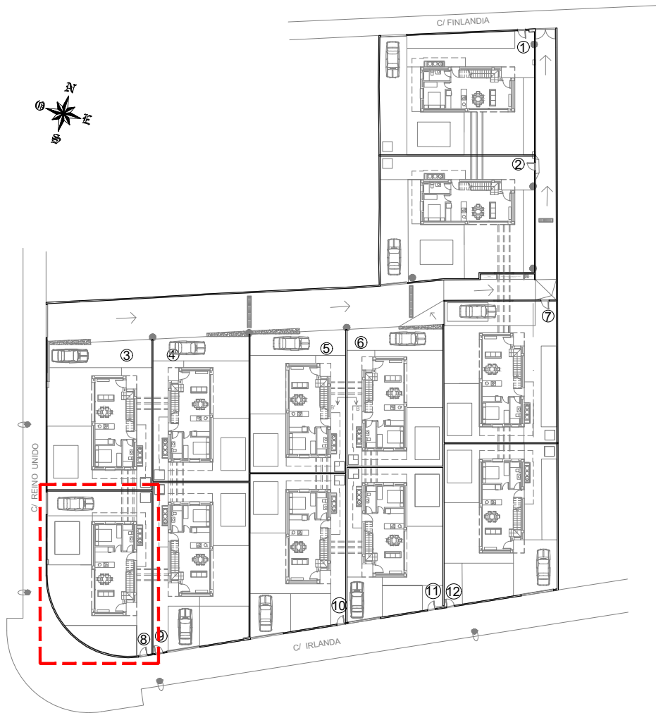
ORDENACIÓN CONJUNTO
