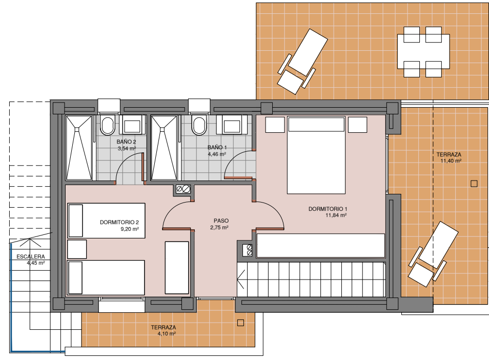
PLANTA ALTA
