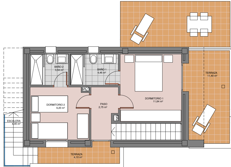
PLANTA ALTA
