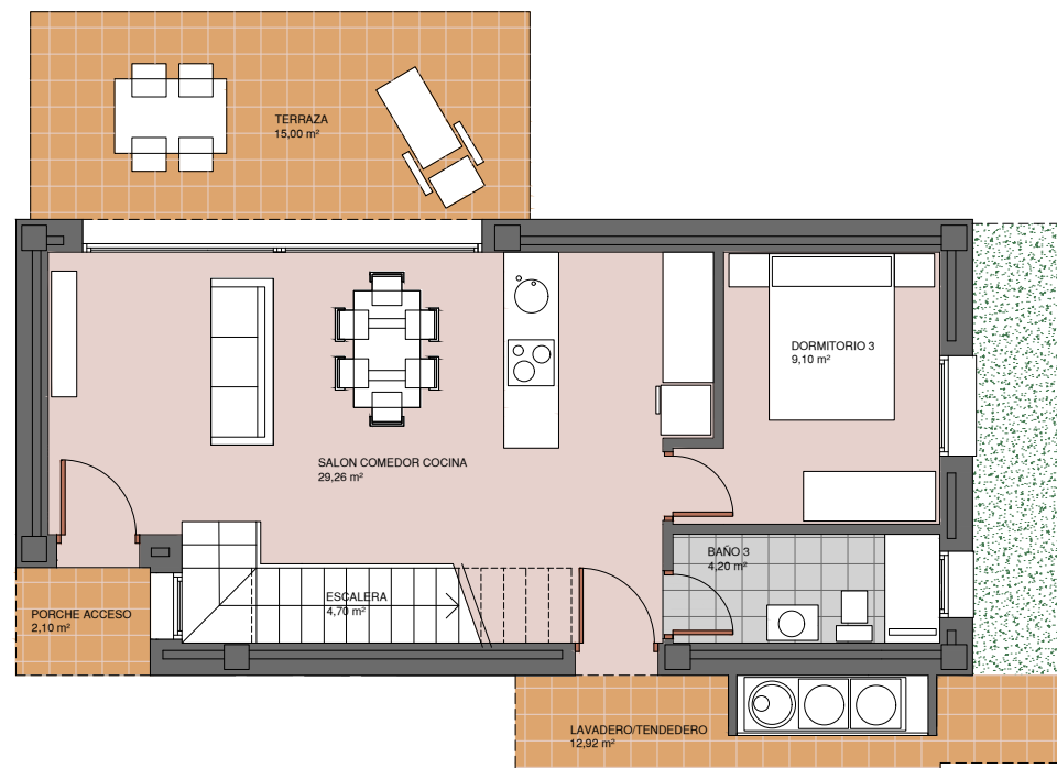
PLANTA BAJA
